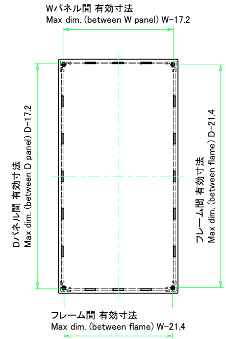
下カバー / Bottom cover
